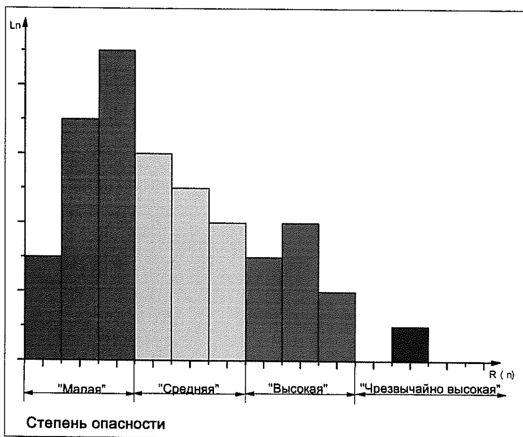
Рис. 16. Иллюстрация формы представления распределения суммарной длины участков L_s трассы по показателю риска аварии R
