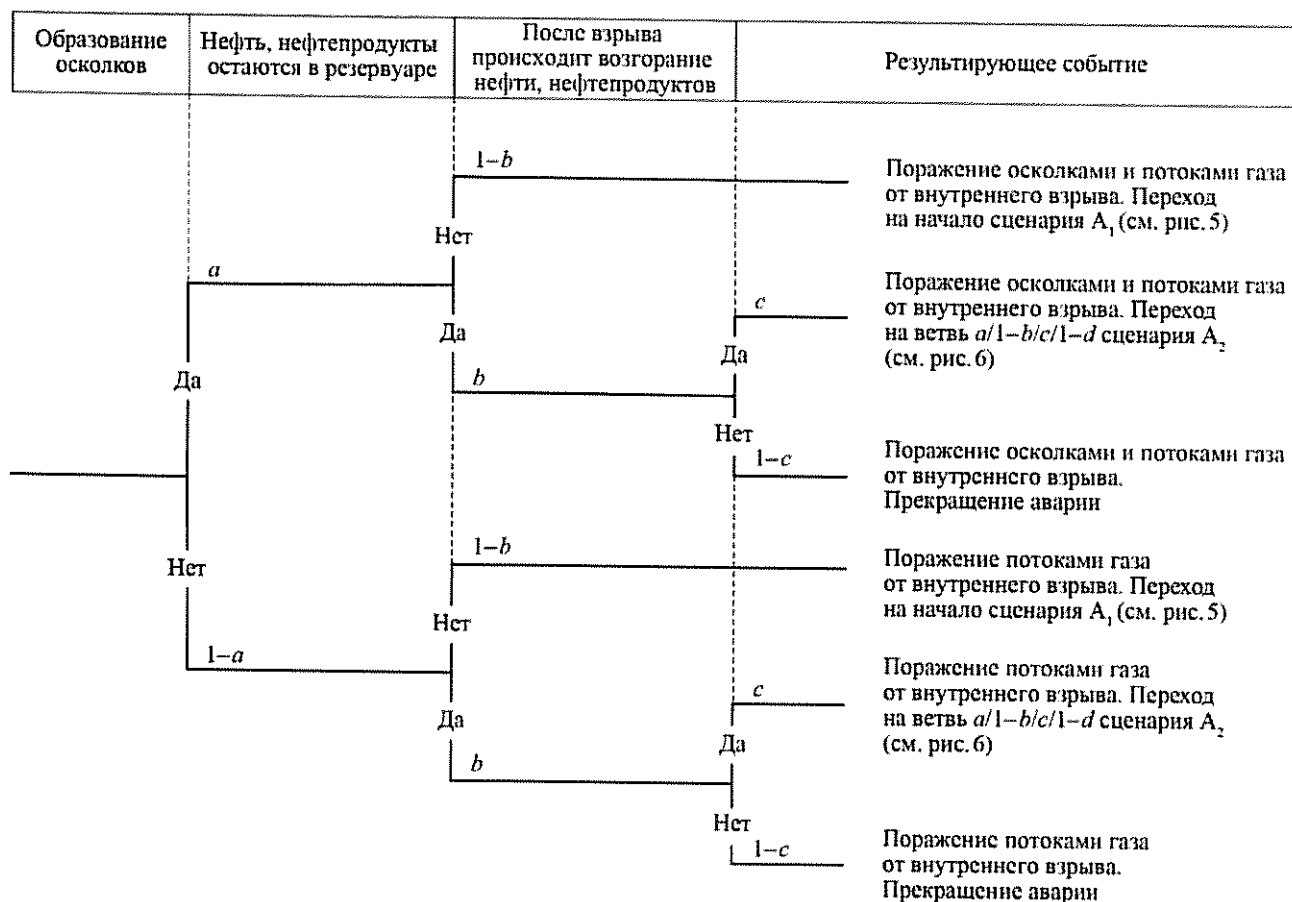
Рис. 7. «Дерево событий» при взрыве внутри наземного резервуара (сценарий A 3 )
