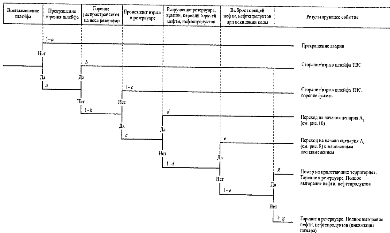
Рис. 9. «Дерево событий» при выходе газовой фазы из подземного резервуара (типа ЖБР) (сценарий A 5 )
