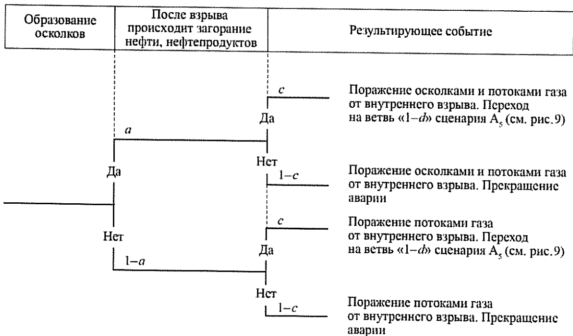
Рис. 10. «Дерево событий» при взрыве внутри подземного резервуара (типа ЖБР) (сценарий A 6 )
